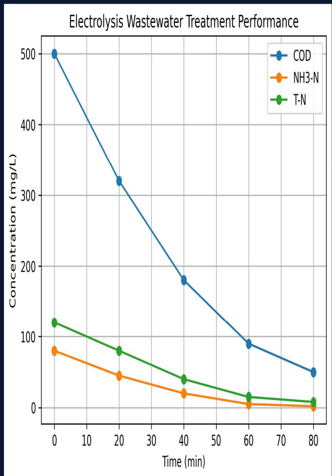
COD, NH 3 -N, T-N 제거 그래프 Removal Performance Graph
